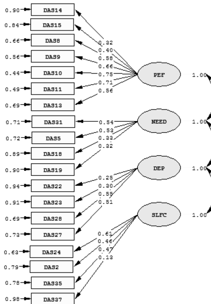
Figure1 Standardized Parameter Estimates DAS-A
